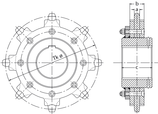
Abbildung 46: HEKO Kettenrad Typ GIA-3, innenverzahnt und austauschbar, für besonders hohe Anforderungen
