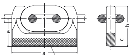
Abbildung 63: HEKO Steckmitnehmer Typ SMO
