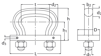
Abbildung 37: HEKO Kettenschloss Typ E
