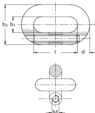
Abbildung 38: Kettenschloss Typ C
