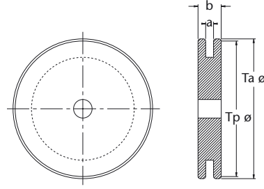
Abbildung 59: HEKO Kettenrad Typ RLE unverzahnt für Laschenketten
