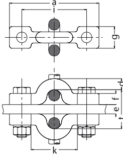
Abbildung 15: Befestigungshälften zur Mitnehmerbefestigung
