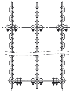
Abbildung 16: Dreistrangkette mit Befestigungshälften
