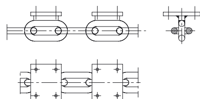
Abbildung 31: Plattenbandförderer als Montageband, offen, zum Beispiel für aufmontiertes Werkzeug
