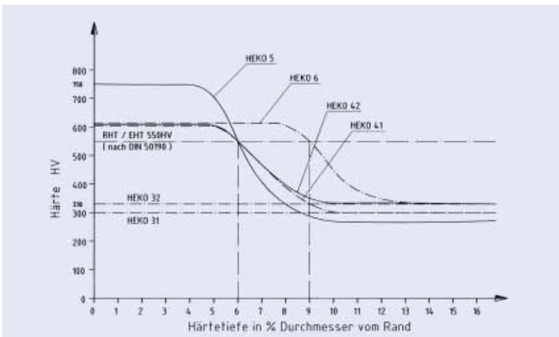
Abbildung 8: Härteverlaufskurven von Befestigungselementen aus Vergütungsstahl in vergüteter und gelenkgehärteter Ausführung sowie einsatzgehärtete Chrom-Nickel legierte Edelstähle
