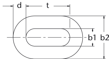
Abbildung 61: HEKO Kettenbügel Typ TS
