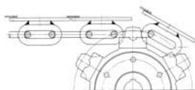
Abbildung 32: Plattenbandförderer als Förderband, geschlossen
