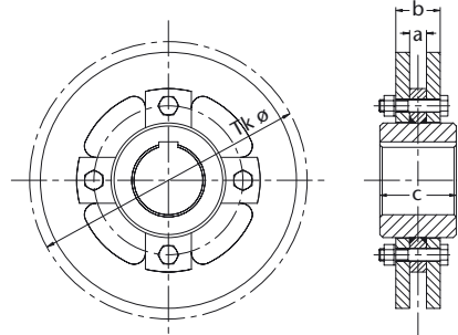
Abbildung 53: HEKO Kettenrad unverzahnt in Stahlausführung Typ GUA – austauschbar
