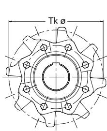
Abbildung 58: HEKO Kettenrad Typ RLA für Gabellaschenkette Modell 69226
