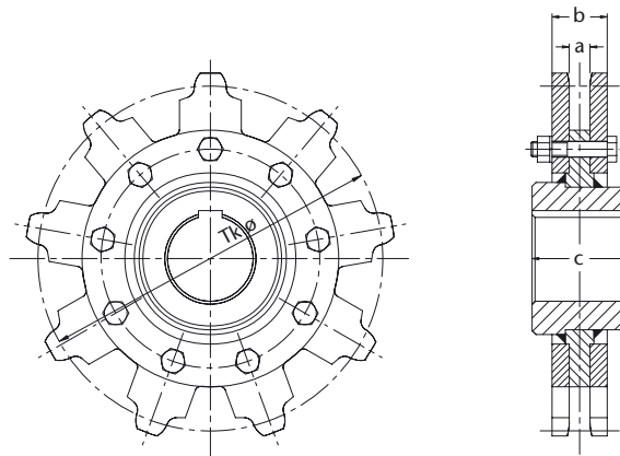
Abbildung 47: HEKO Kettenrad Typ GTA, taschenverzahnt, austauschbar, Nabe in geschweißter Ausführung
