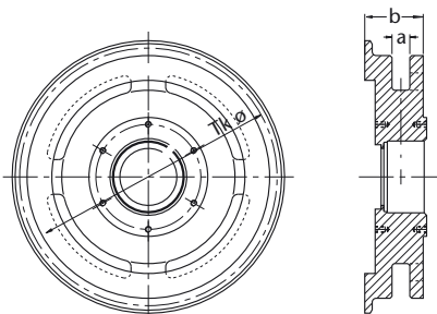
Abbildung 67: HEKO Stützrollen Typ VUE aus Stahl in gedrehter Ausführung
