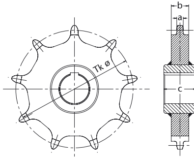
Abbildung 42: HEKO Kettenrad Typ VIE-B einteiliges, innenverzahnung, geschweißtes Kettenrad mit mechanisch bearbeiteter Kettenauflage Nabe aus Stahl, Zahnkranz aus legiertem CrMo-Stahl
