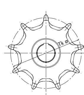
Abbildung 43: HEKO Kettenrad Typ VIE-C und VIE-D mit angeschrägten Ausfallöffnungen – aus dem Vollen gedreht bzw. in geschweißter Ausführung (alternativ zu VIE-A und VIE-B)
