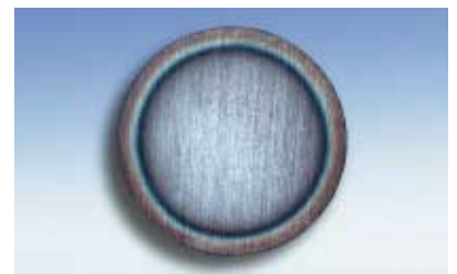
Abbildung 4: Querschnitt durch ein einsatzgehärtetes Kettenglied.
