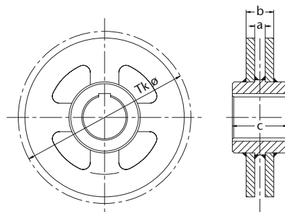
Abbildung 54: HEKO Kettenrad unverzahnt in Stahlausführung Typ GUE – einteilig
