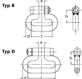
Abbildung 36: Kettenschloss Typ B mit angeschweißter Mutter, Typ D mit loser Mutter
