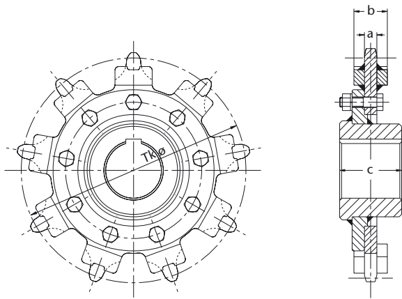
Abbildung 44: HEKO Kettenrad Typ GIA, innenverzahn- tes austauschbares Kettenrad mit angeschweißter Kettenauflage
