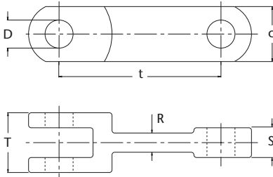
Abbildung 55: HEKO Gabellaschenkettens, gesenkgeschmiedet, Einzelstrang
