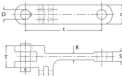
Abbildung 56: HEKO Gabellaschenkettens, gesenkgeschmiedet, Doppelstrang
