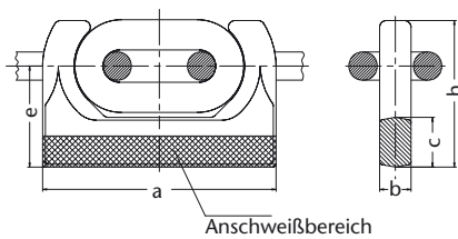
Abbildung 19: HEKO Steckmitnehmer SMO
