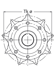
Abbildung 57: HEKO Kettenrad Typ RLA-R mit symmetrischen Zähnen für Reversierbetrieb
