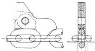
Abbildung 33: Mitnehmer mit Ausklinkvorrichtung für Reversierbetrieb
