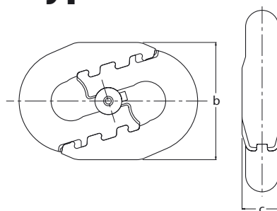
Abbildung 39: HEKO Kettenschloss Typ FL
