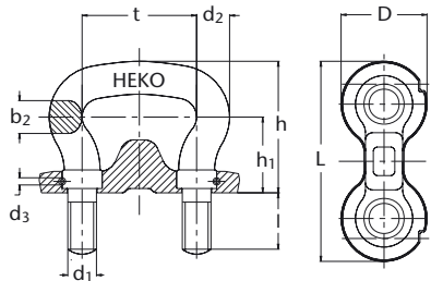
Abbildung 11: HEKO Kettenbügel Typ TS
