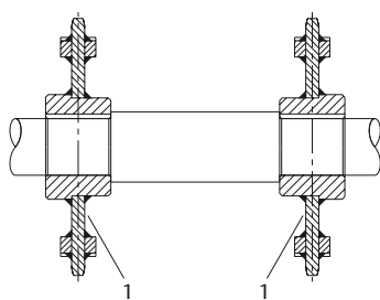
Abbildung 68: Montagehinweis 1
