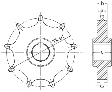
Abbildung 41: HEKO Kettenrad Typ VIE-A innenverzahnung, einteiliges Kettenrad mit mechanisch bearbeiteter Kettenauflage komplett aus legiertem CrMo-Stahl
