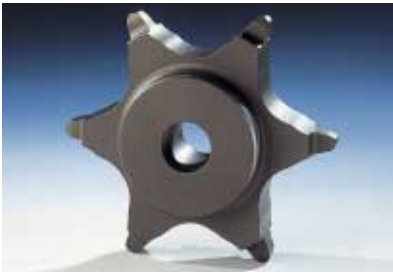
Abbildung 41: HEKO Kettenrad Typ VIE-A innenverzahnung, einteiliges Kettenrad mit mechanisch bearbeiteter Kettenauflage komplett aus legiertem CrMo-Stahl
