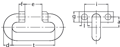
Abbildung 21: HEKO Befestigungsglieder Typ BGQ
