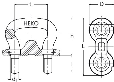
Abbildung 61: HEKO Kettenbügel Typ TS
