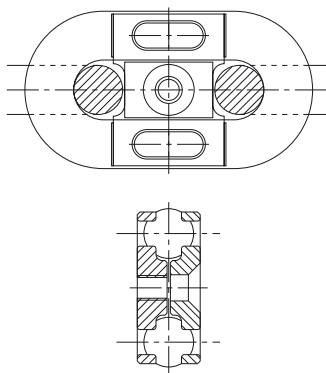
Abbildung 35: Kettenschloss Typ F
