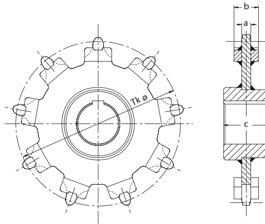
Abbildung 45: HEKO Kettenrad Typ GIE, innenverzahntes, einteiliges Kettenrad mit angeschweißter Kettenauflage
