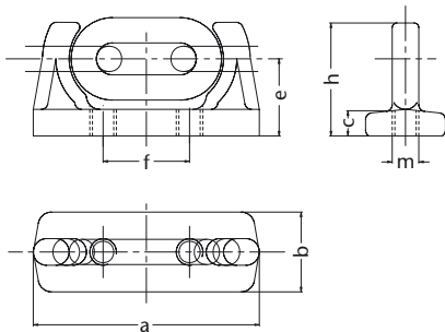
Abbildung 18: HEKO Steckmitnehmer SMG
